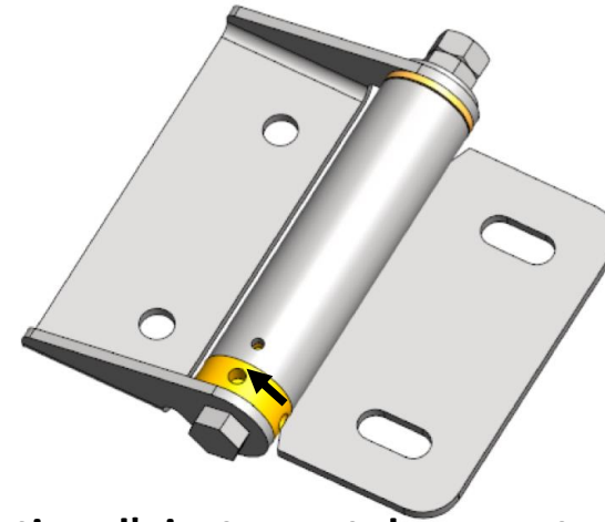
Direction d'ajustement du ressort
